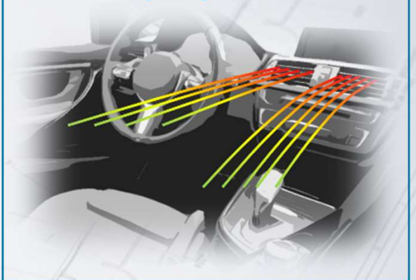
Durchströmung Fahrgastzelle
